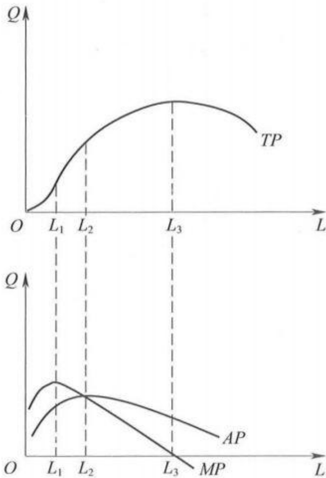
图 3-1 生产函数图形及其位置关系
